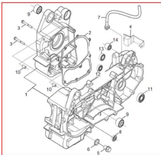
CARCAÇAS DO MOTOR
